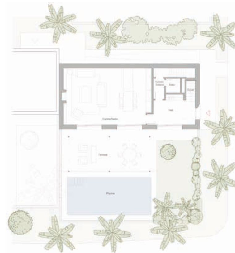
Planta Baja
