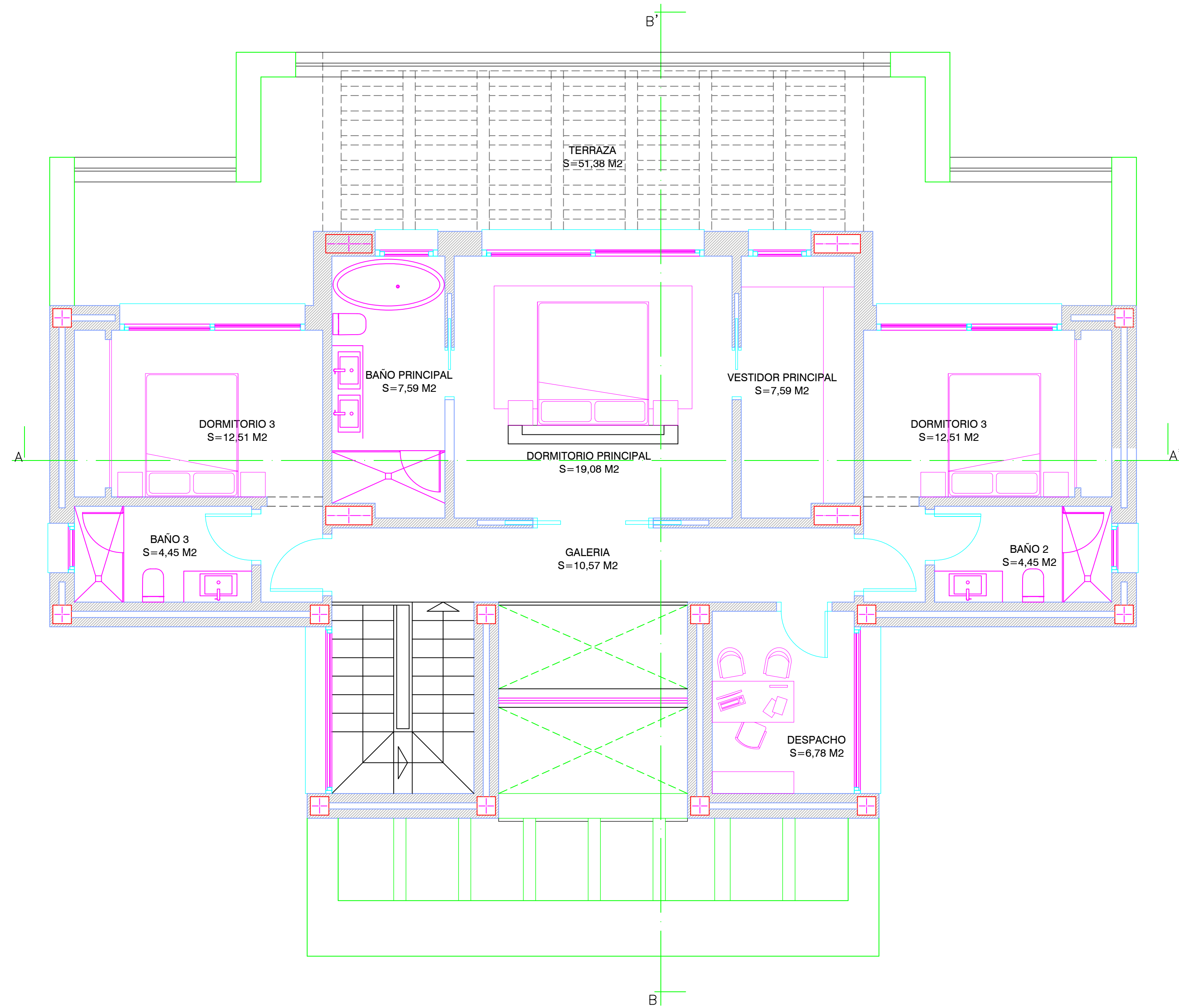
PLANTA ALTA
