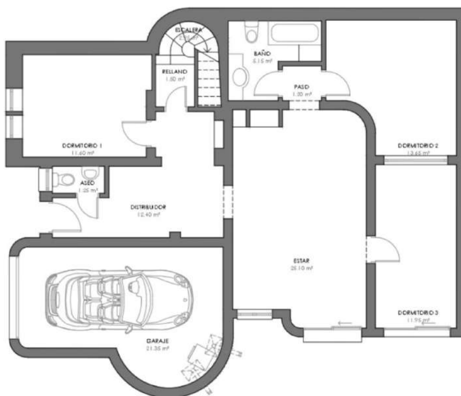
DISTRIBUCION PLANTA SEMISÓTANO
