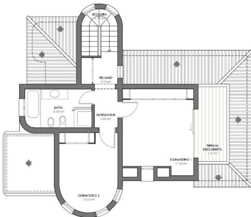
DISTRIBUCION PLANTA ALTA
