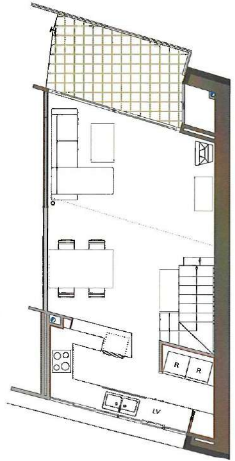
PLANTA PRIMERA
