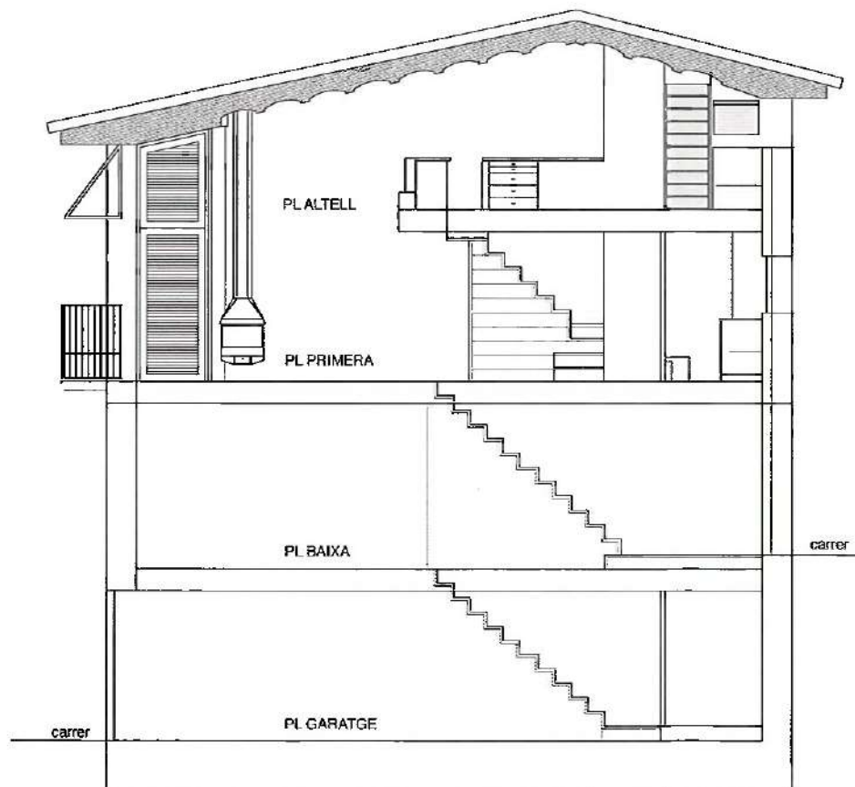
SECCIÓ
