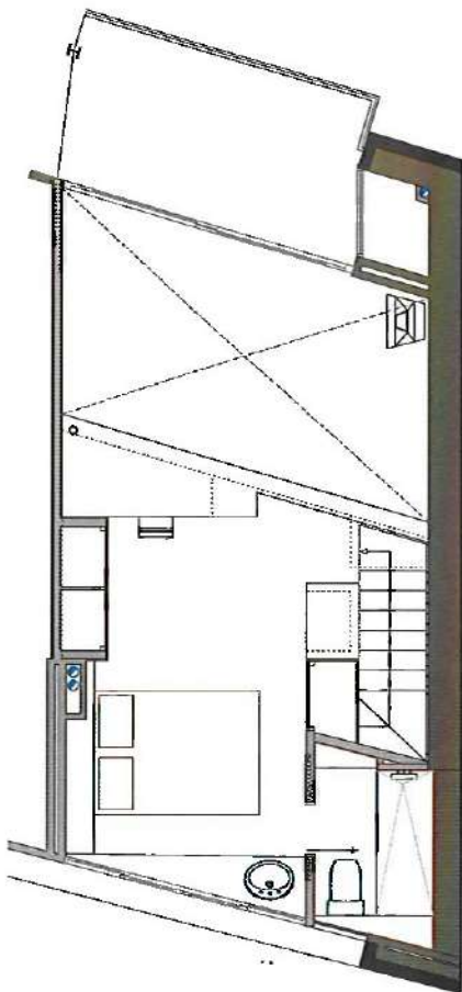
PLANTA ALTELL
