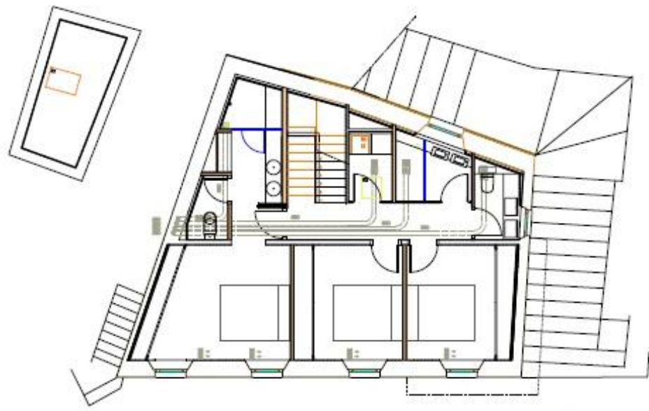
Planta inferior
