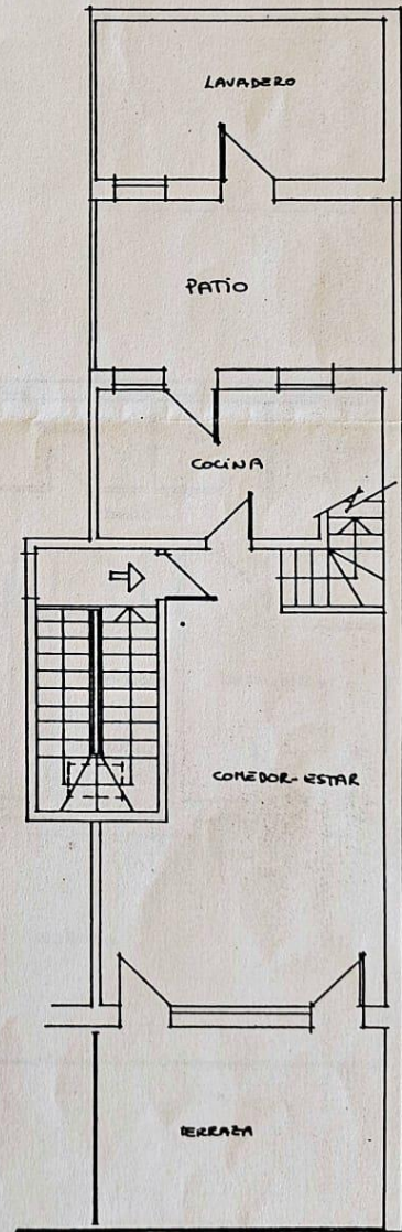
PLANTA PRIMERA
