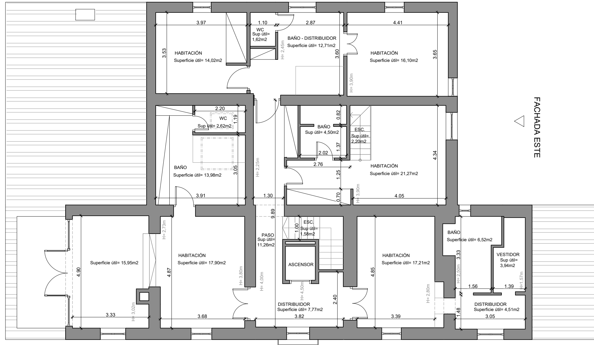
PLANTA PRIMERA Superficie útil=175,66m2
