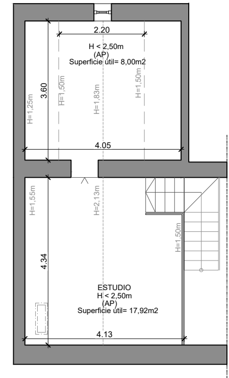
PLANTA ALTILLO Superficie útil=25,92m2
