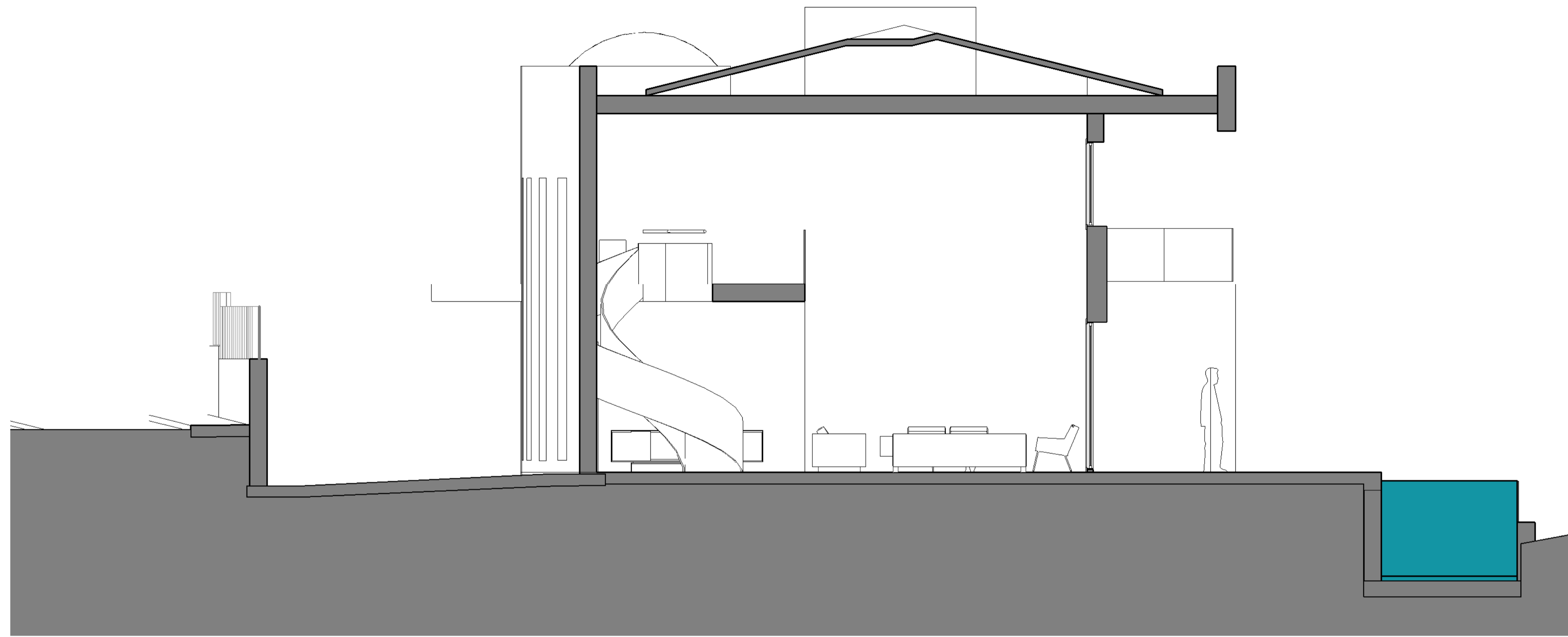
2 imp secció transversal A104 1:50
