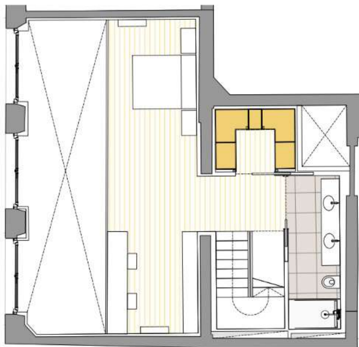
PLANTA ALTILLO 51.83 m²
