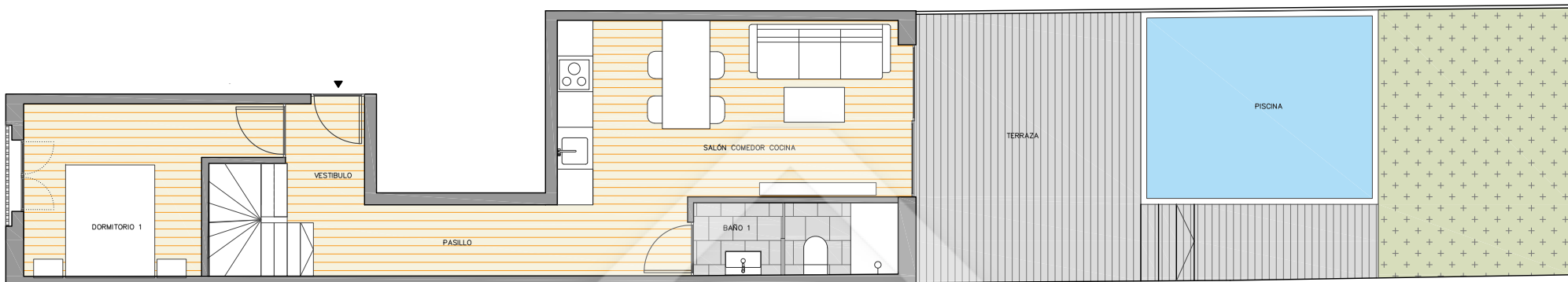
PLANTA BAJA
