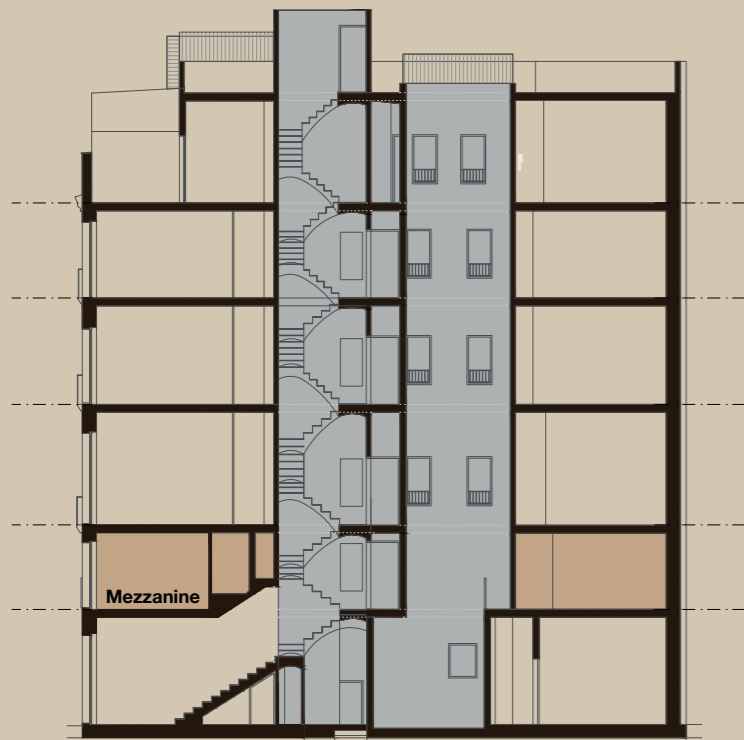
SECTION / SECCIÓN
