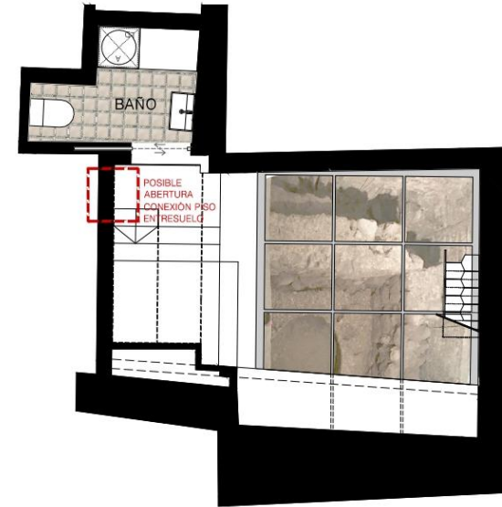
PLANTA SÓTANO
