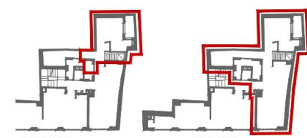
C/ SAN SEVER PLANTA SÓTANO
