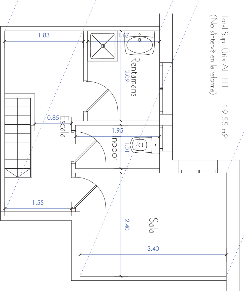
PLANTA DE L'ALTELL | Cotes
