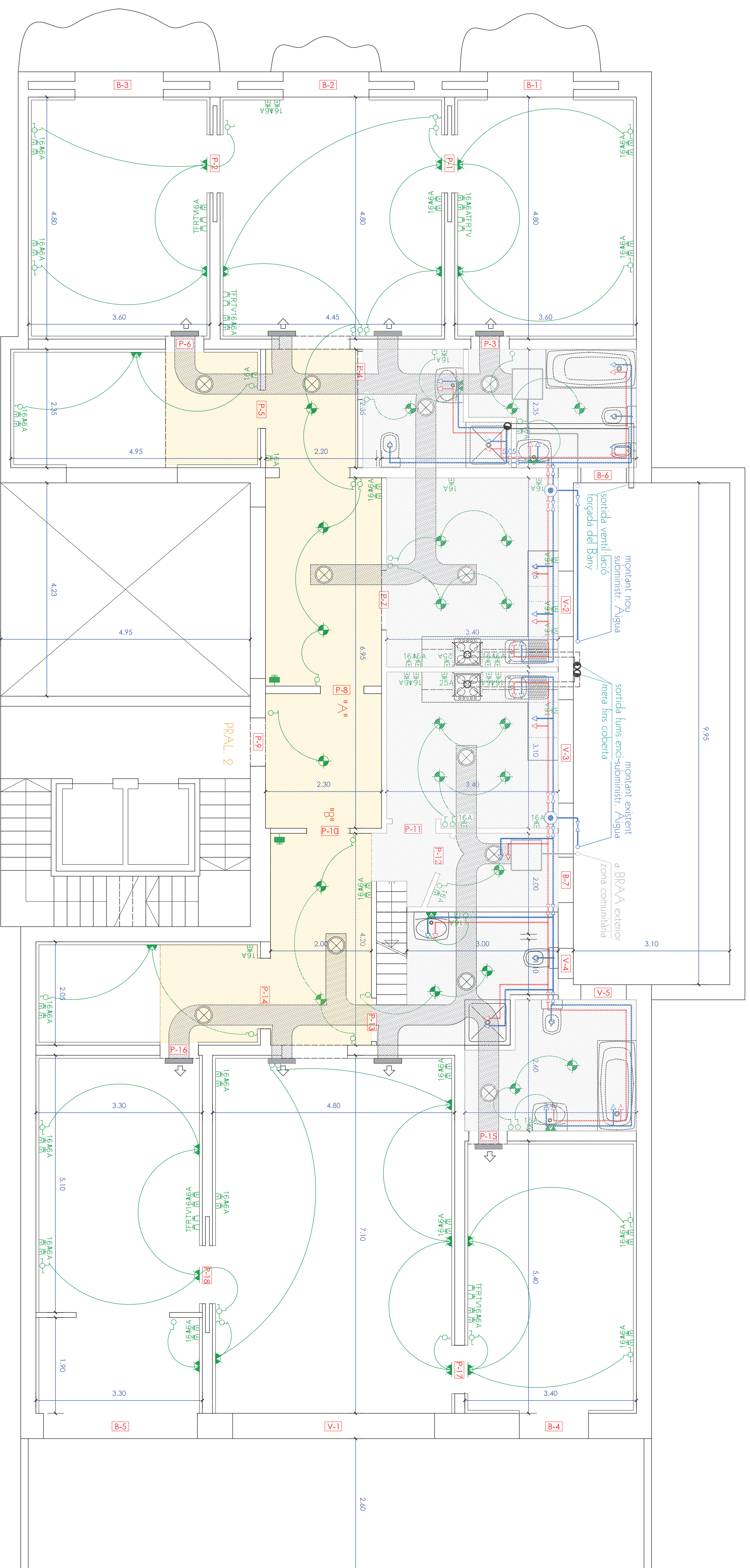
PLANTA DE LES INSTAL·LACIONS | Cotes
