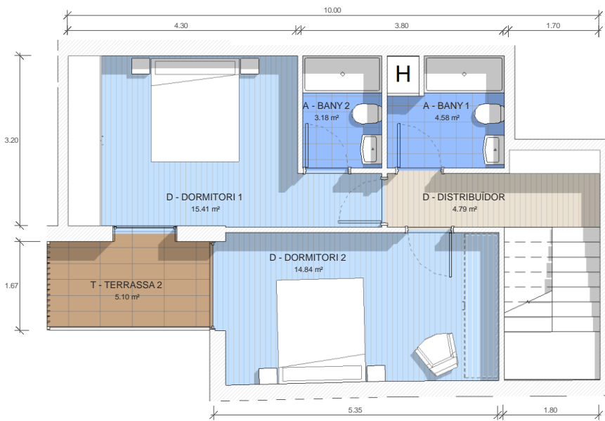
PLANTA PRIMERA
