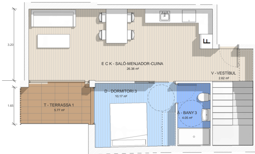
PLANTA SEGONA
