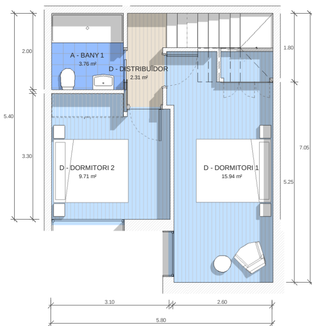
PLANTA PRIMERA
