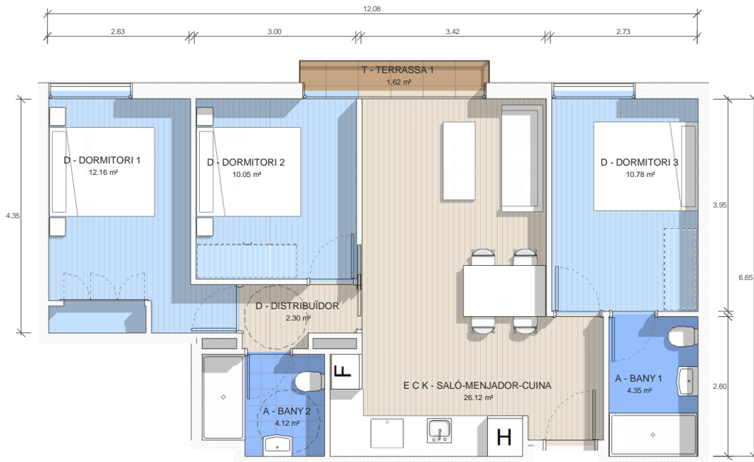
PLANTA SEGONA
