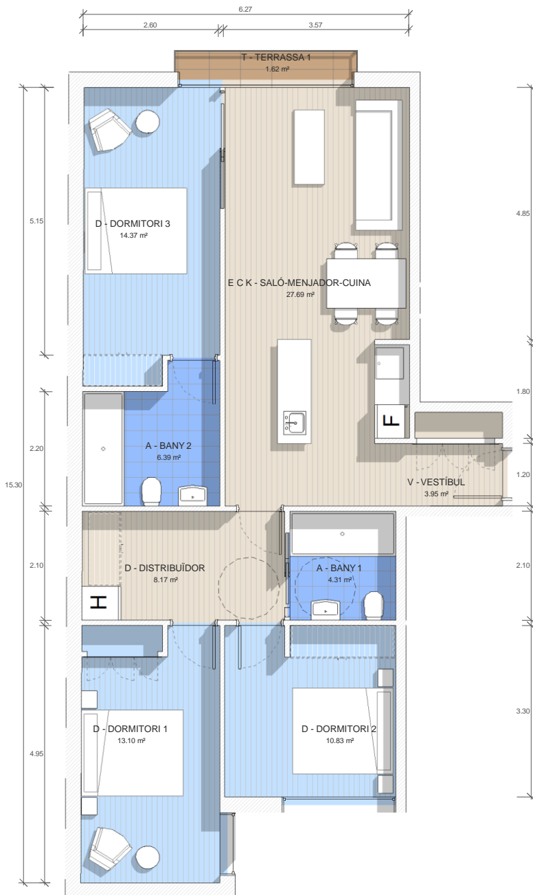
PLANTA PRIMERA
