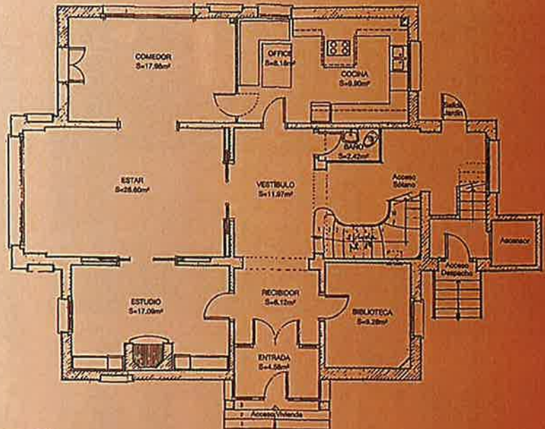
Planta Baja
