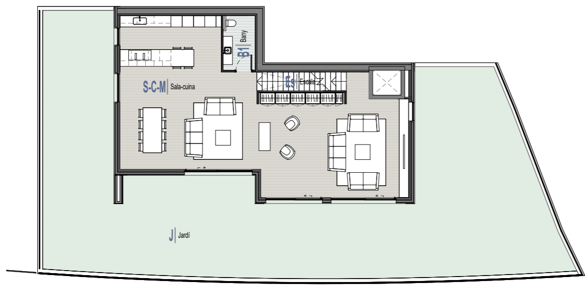
Planta Baixa 1 : 200
