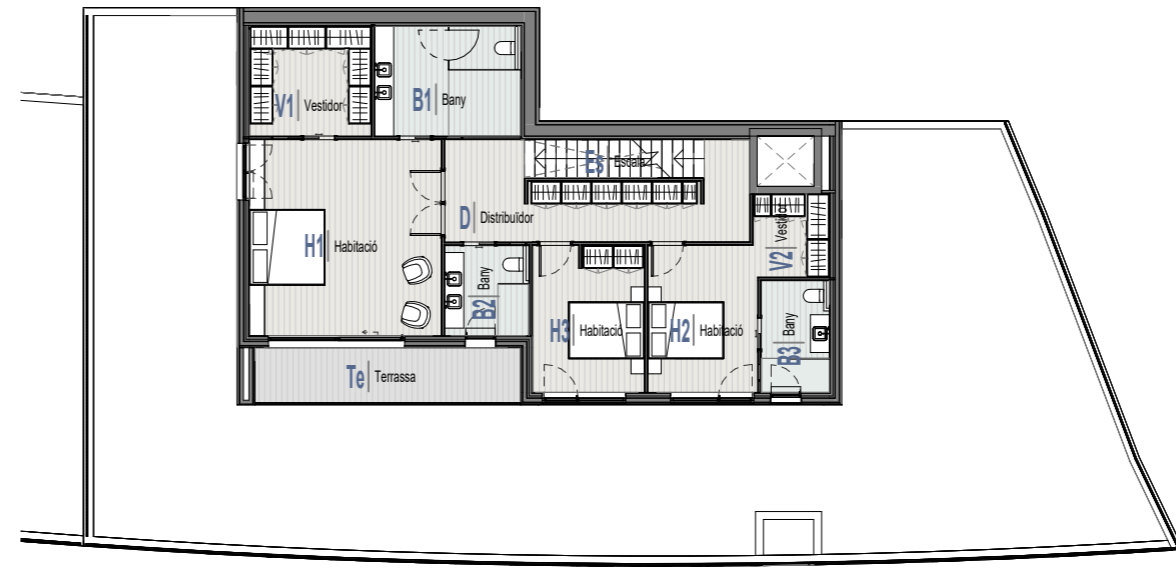
Planta Primera 1 : 200
