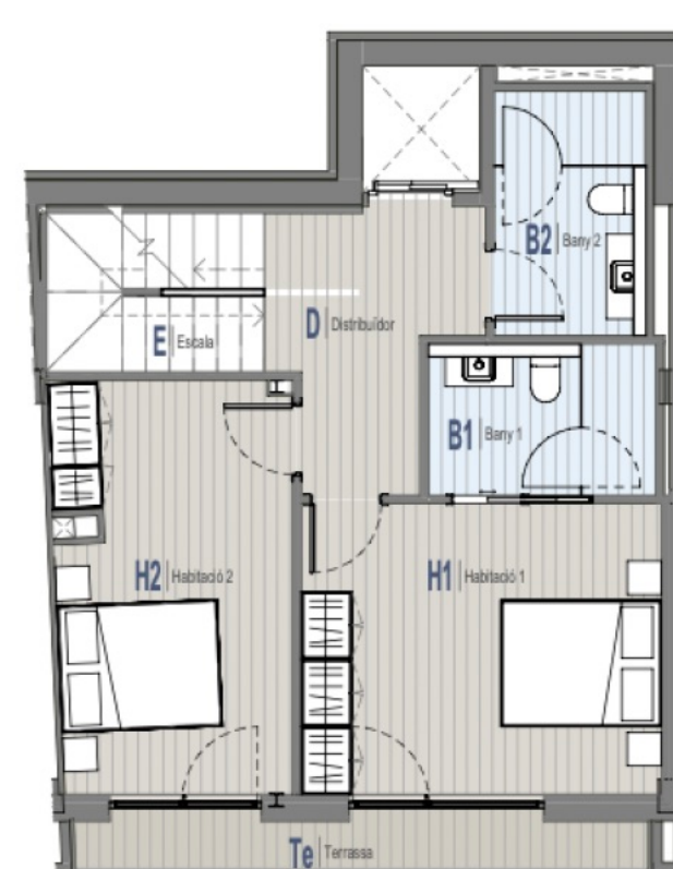
3 Planta Primera 1 : 100
