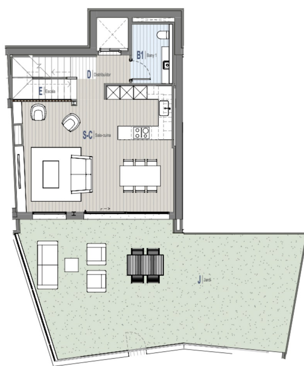
2 Planta Baixa 1 : 100
