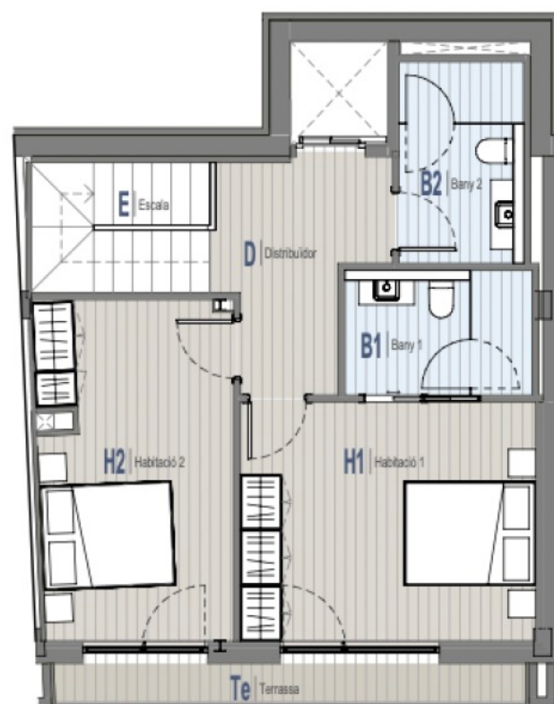
4 Planta Sotacoberta 1 : 100
