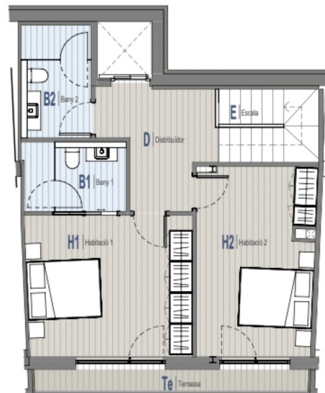
4 Planta Sotacoberta 1 : 100
