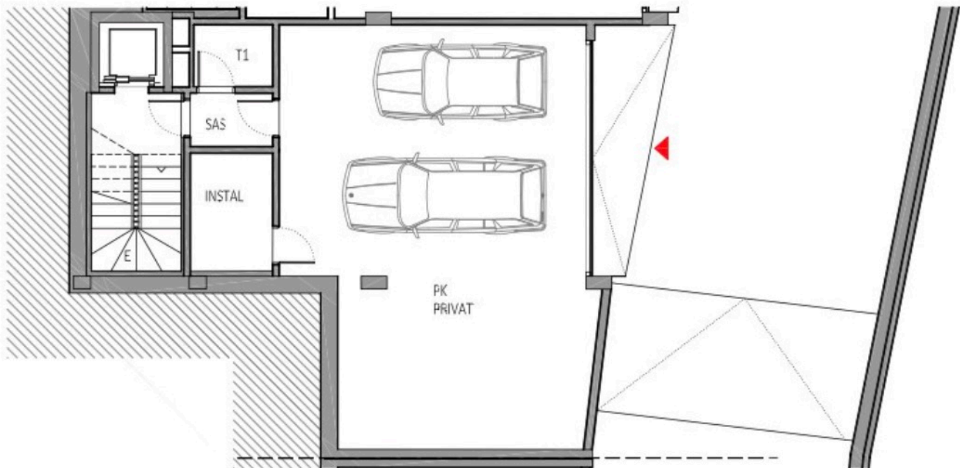
PLANTA SOTERRANI
