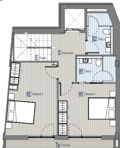
3 Planta Primera 1 : 100
