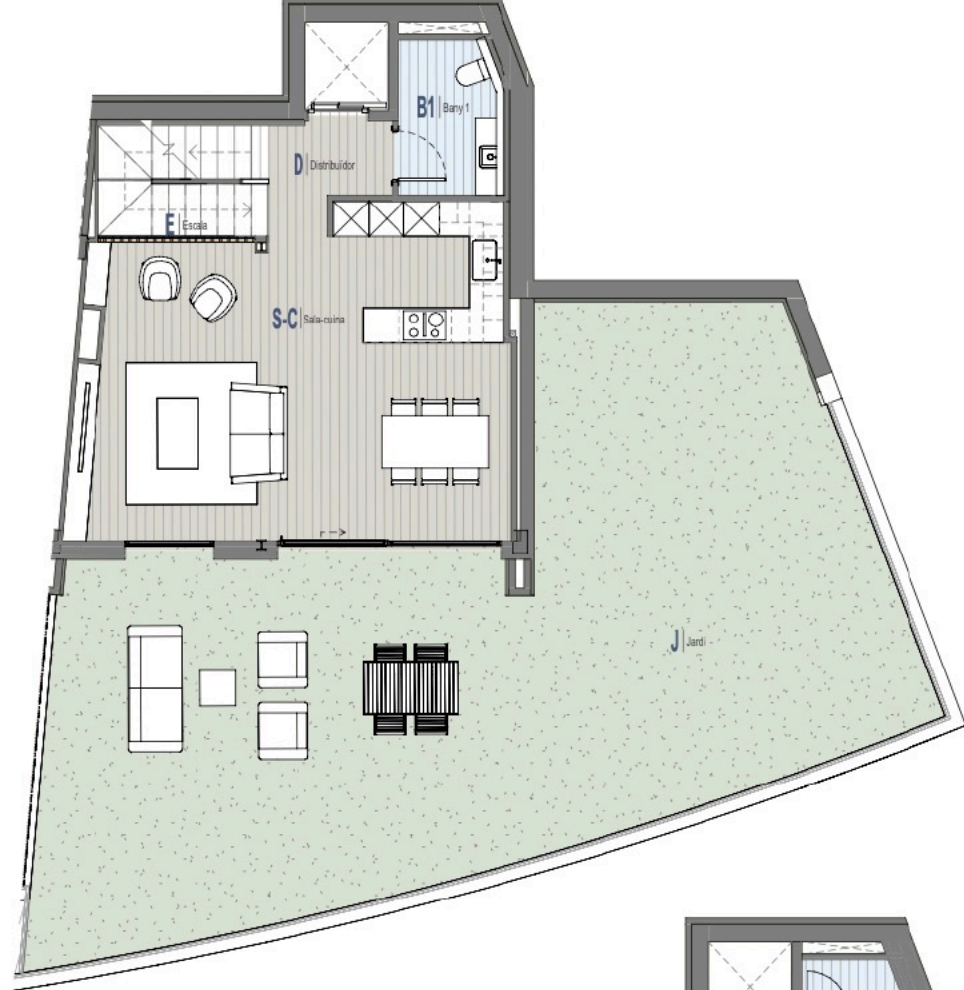
2 Planta Baixa 1 : 100
