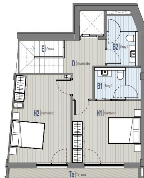
4 Planta Sotacoberta 1 : 100
