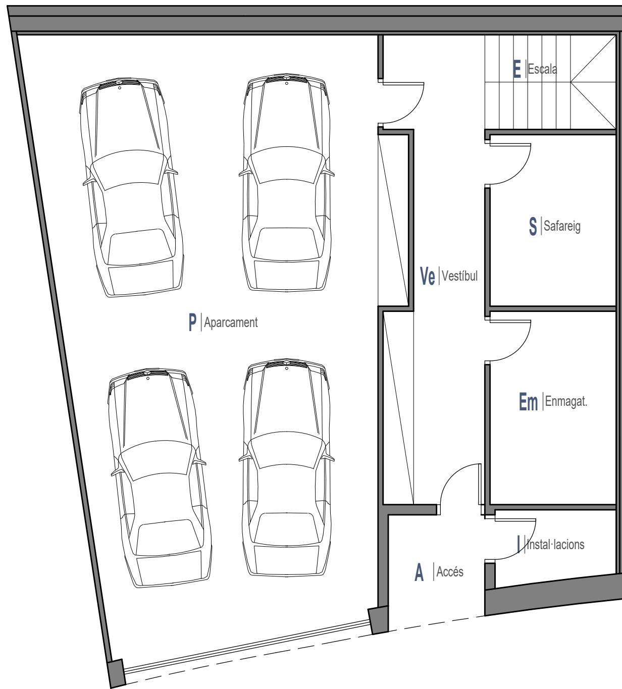
P. Soterrani - Distribució Arq 1 : 75
