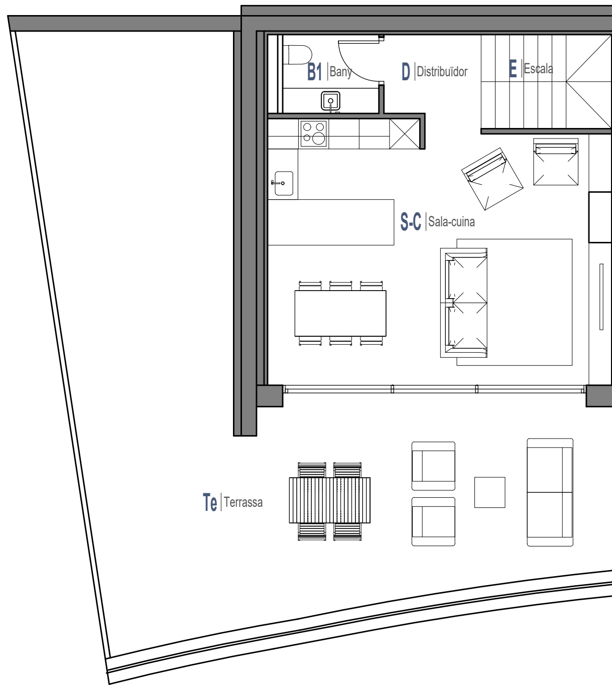
P. Baixa - Distribució Arq 1 : 75
