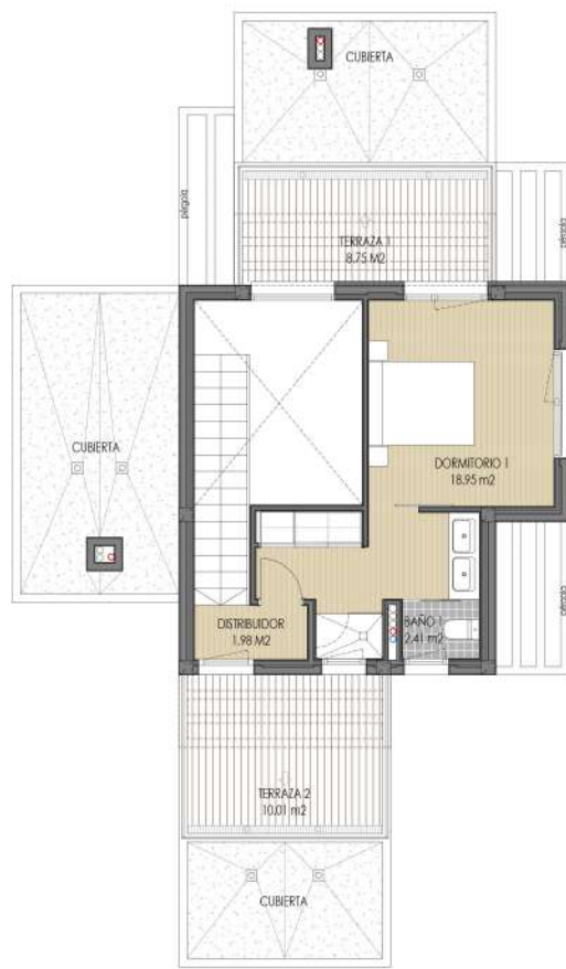
PLANTA PRIMERA
