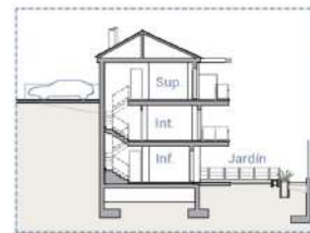
Sección / Section
