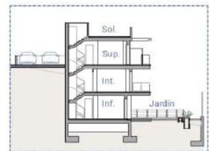
Sección / Section
