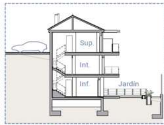
Sección / Section
