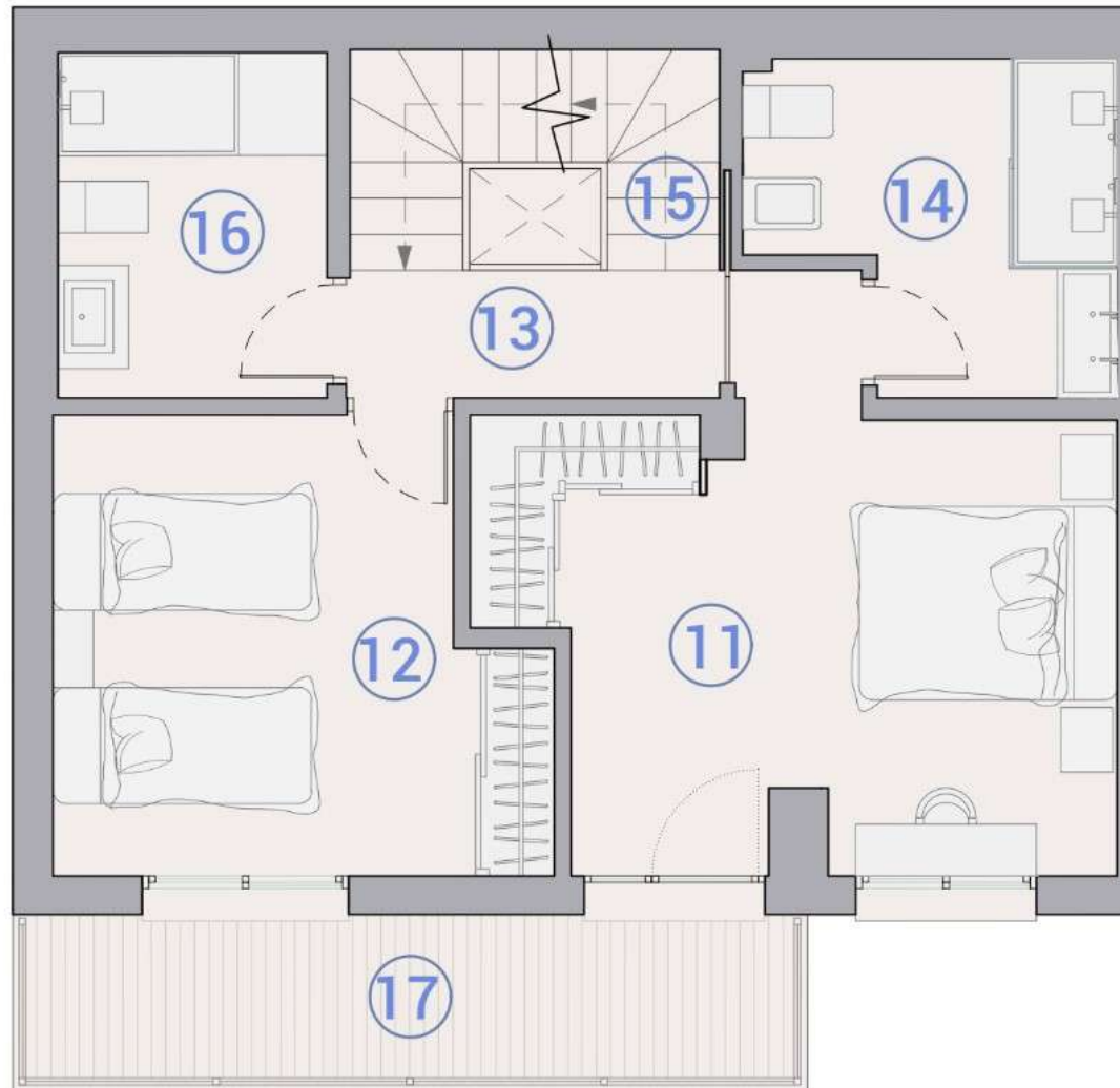
Planta / Floor Intermedia
