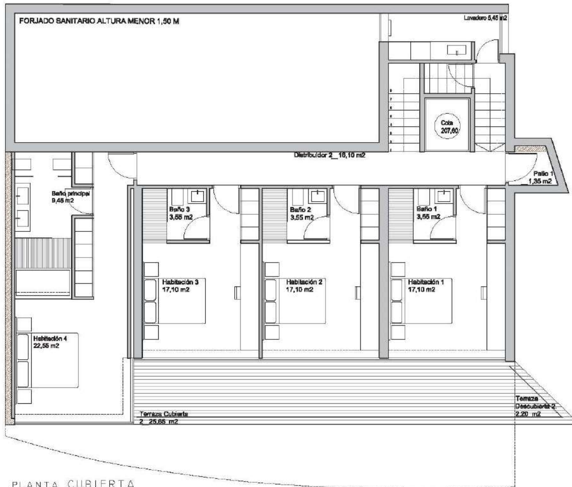
PLANTA CUBIERTA ESCALA 1 - 200
