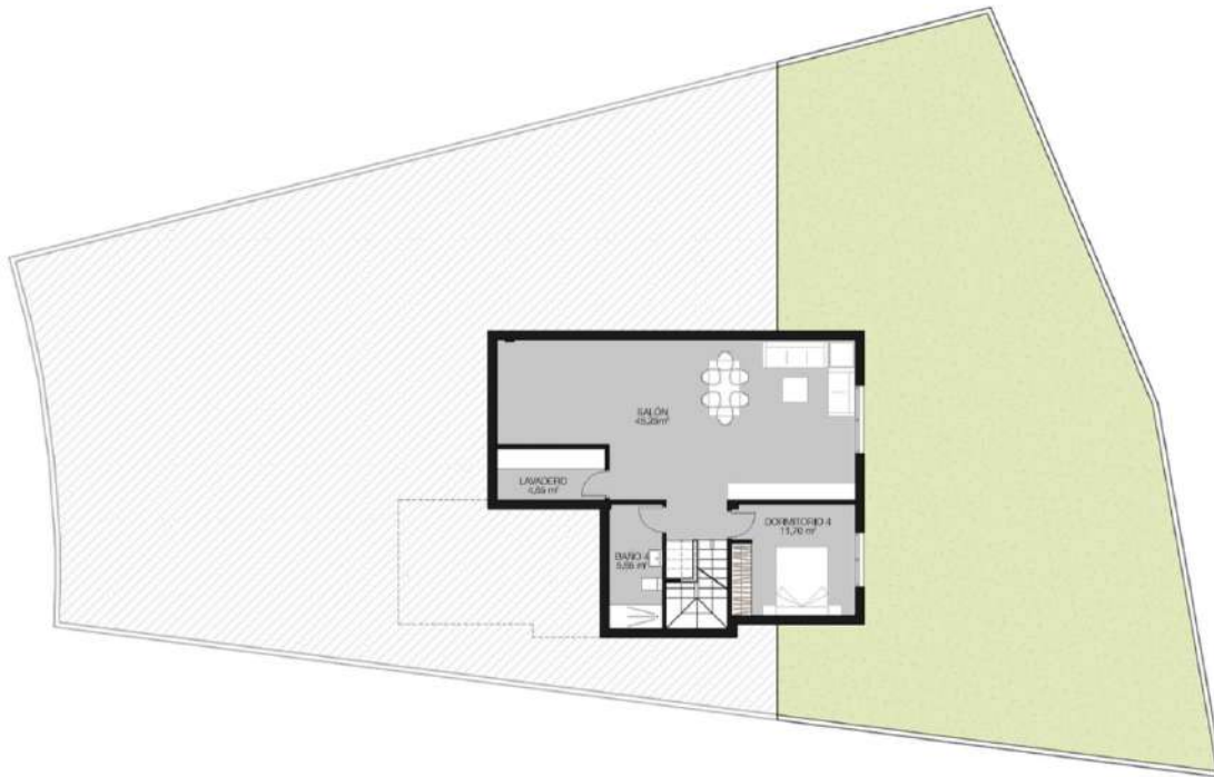
PLANTA SOTANO/ BASEMENT SUP. CONSTRUIDA: 83,26 m 2
