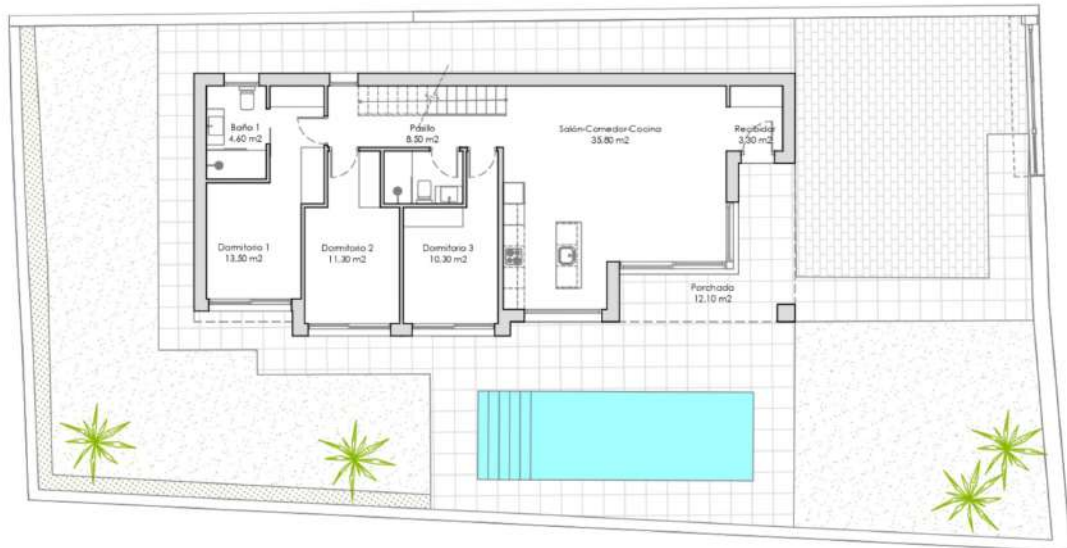
PLANTA BAJA
