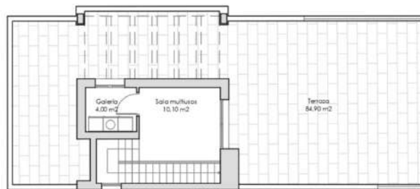
PLANTA PRIMERA
