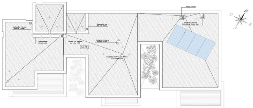
Planta Cubierta
