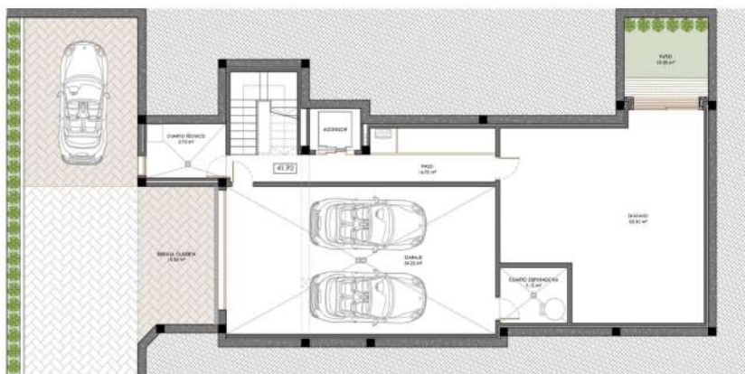
Planta Sótano
