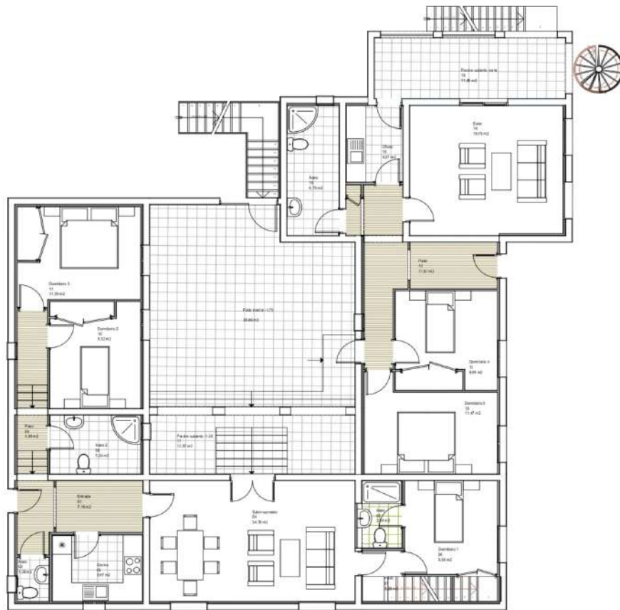
0. PLANTA BAJA 1:100
