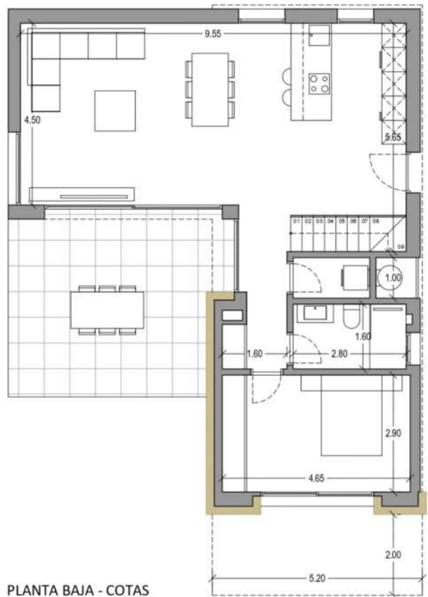
PLANTA BAJA - COTAS
