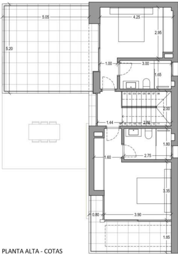
PLANTA ALTA - COTAS
