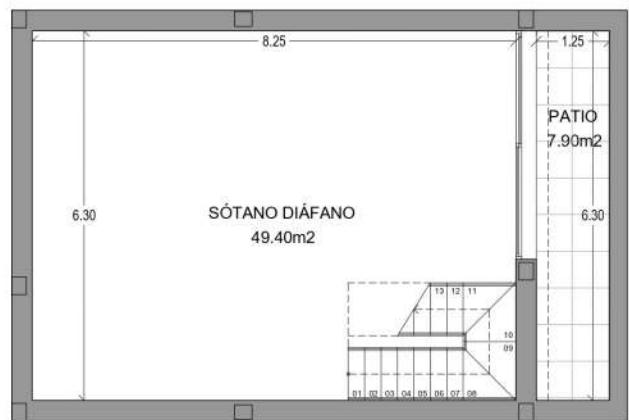
SÓTANO - SUPERFICIES Y COTAS
