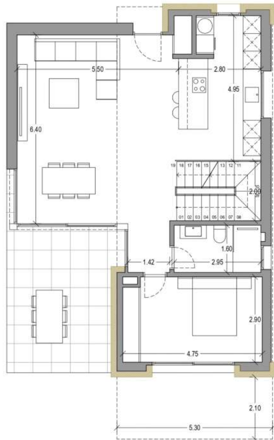
PLANTA BAJA - COTAS
