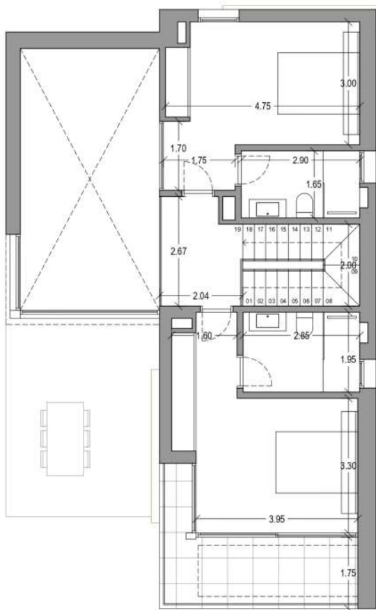
PLANTA ALTA - COTAS
