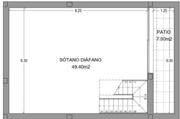
SÓTANO - SUPERFICIES Y COTAS
