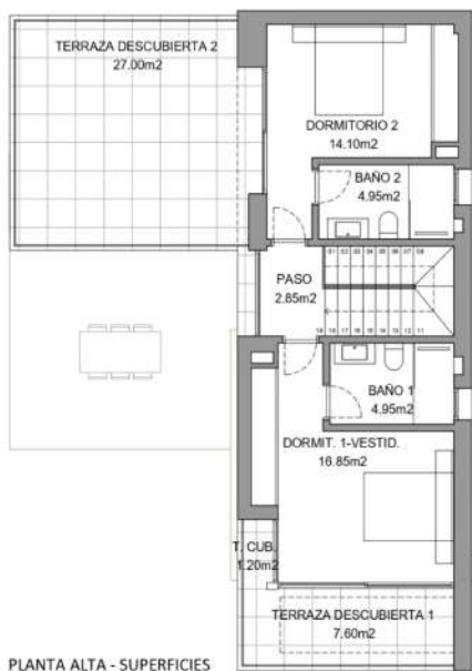
PLANTA ALTA - SUPERFICIES
