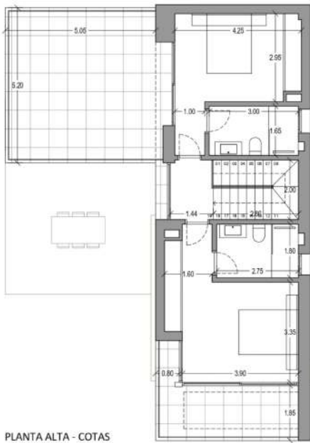
PLANTA ALTA - COTAS
