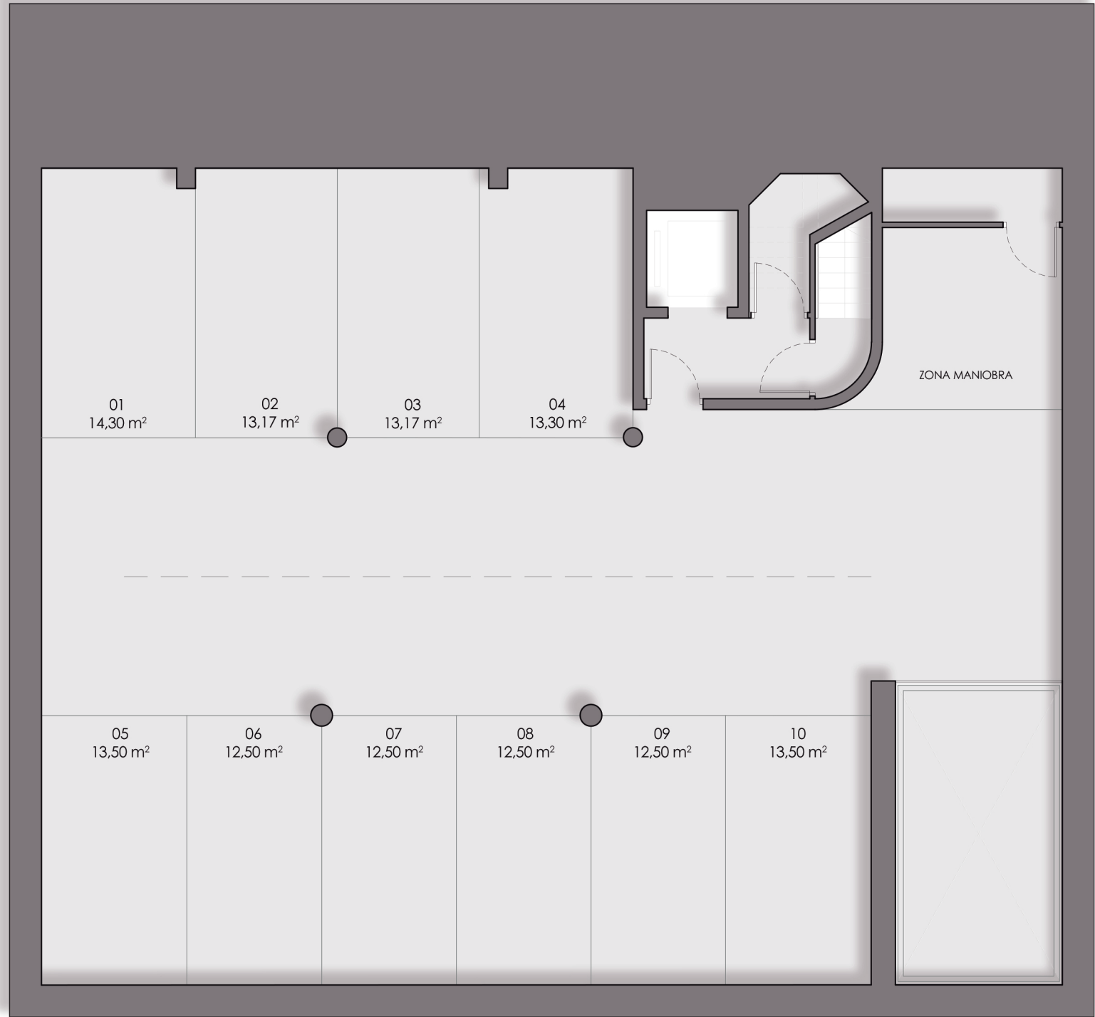
GARAJE - PLANTA SOTANO
