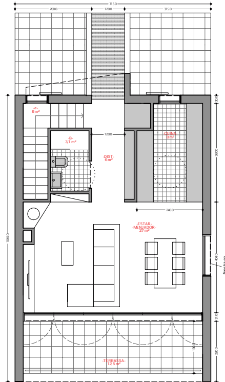
Planta Primera
