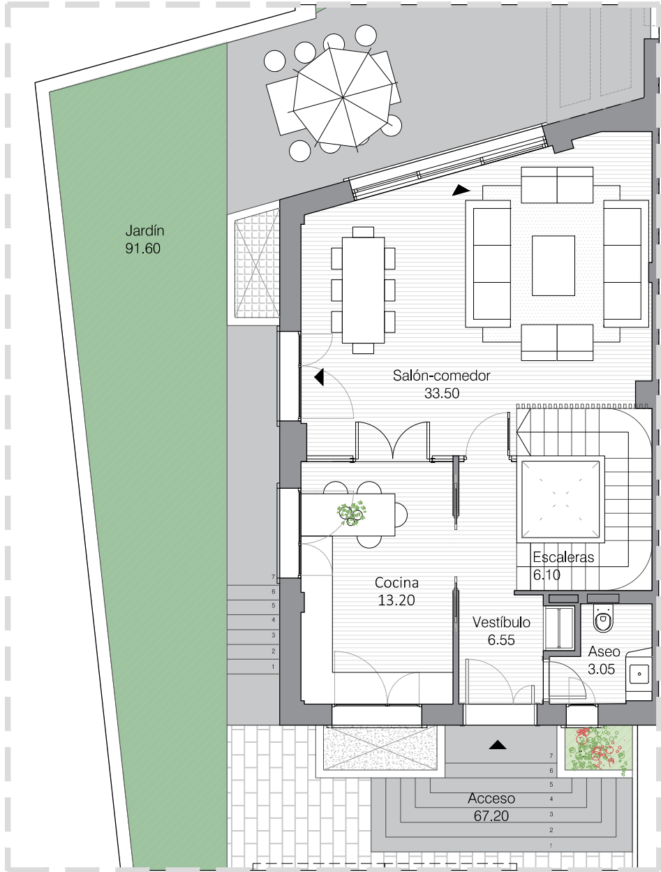
PLANTA BAJA
