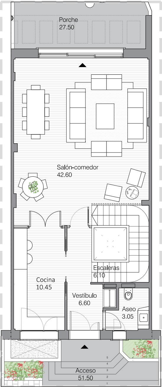
PLANTA BAJA
