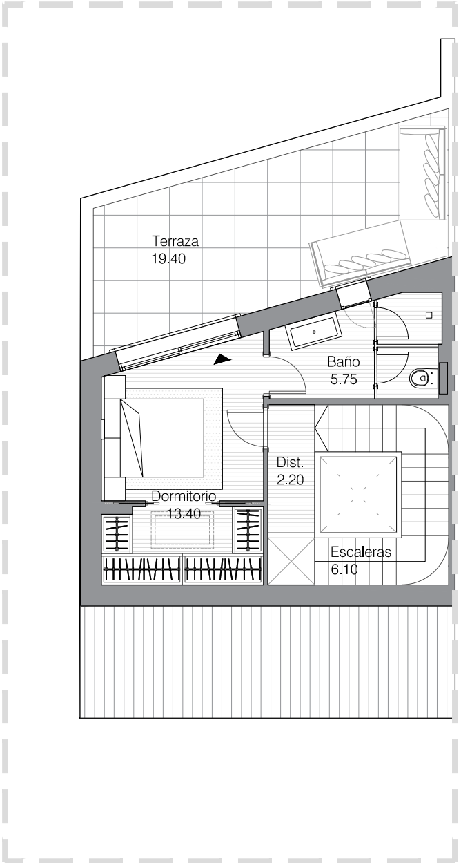
PLANTA ÁTICO
