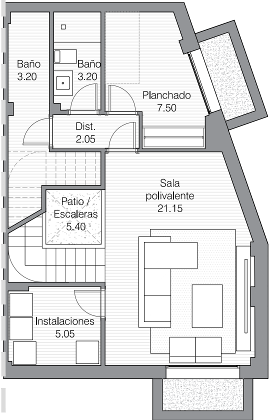
PLANTA SÓTANO
