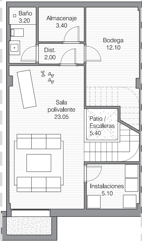
PLANTA SÓTANO
