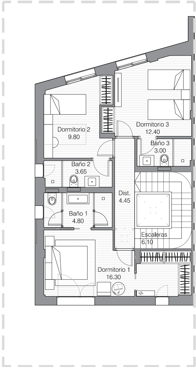
PLANTA PRIMERA
