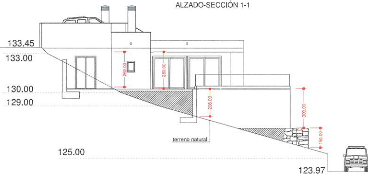
ALZADO-SECCIÓN 1-1
