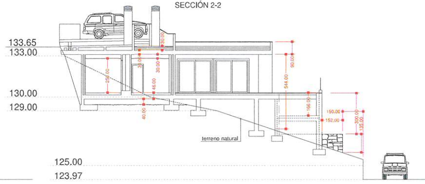
SECCIÓN 2-2
