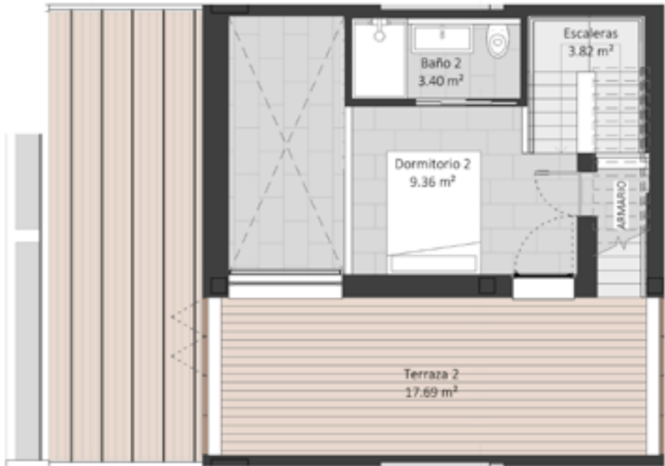
Planta Primera / FIRST FLOOR
